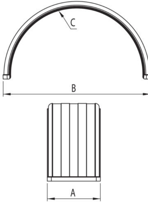
Çamurluk Kanallı Mudguard
