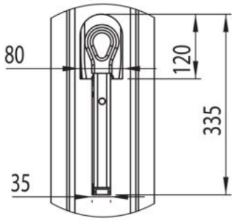
DETAY B ÖLÇEK 1:10
